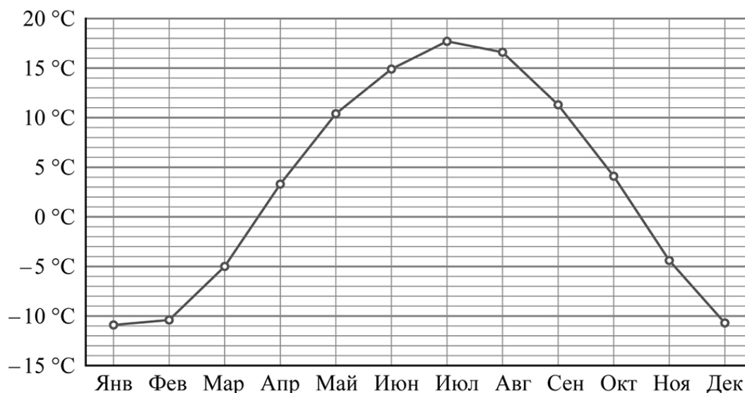
Средняя температура воздуха в Эдмонтоне по месяцам
