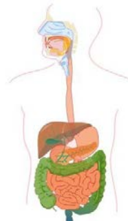
Пищеварительная система
